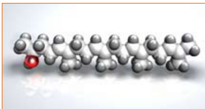
Geranylgeranylpropanol (GGP)
