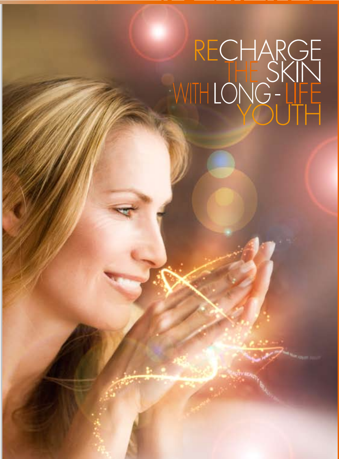
Geranylgeranylpropanol (GGP)
